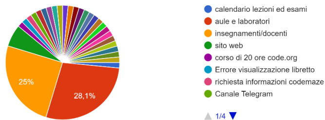
Figura 4. Distribuzione argomenti
